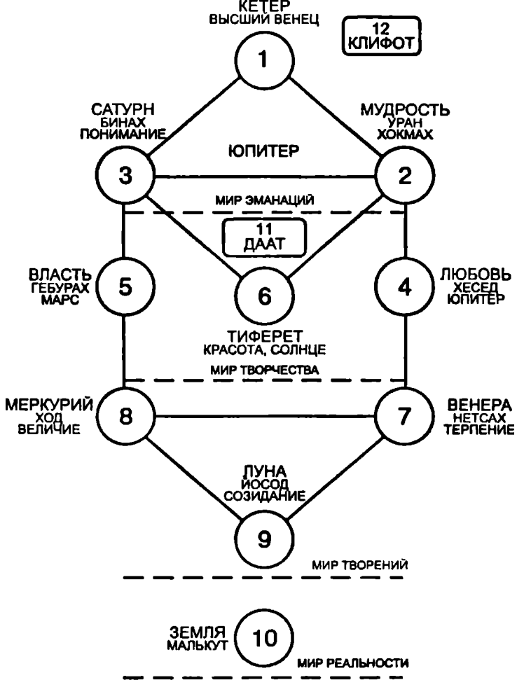
Рис. 2. Древо Сефирот
